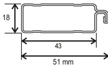
Rozměr profilu dveřní sítě
